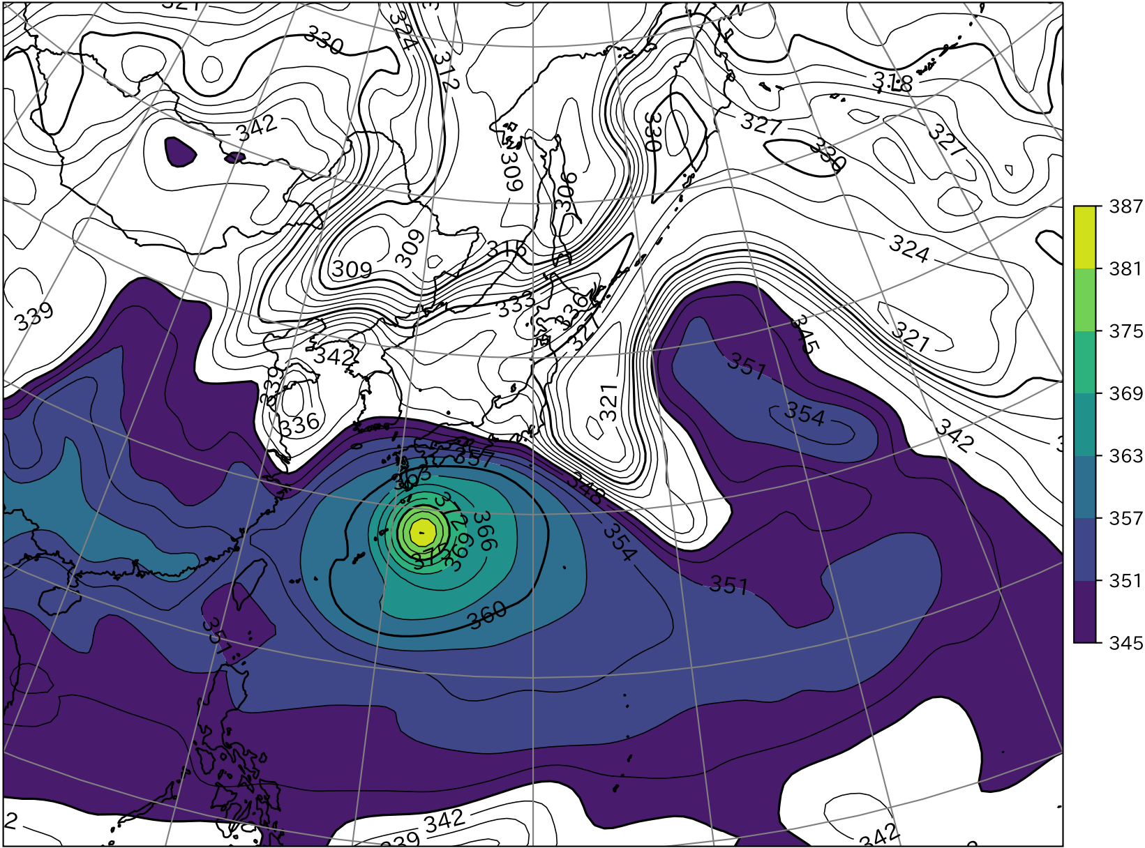
850hpa 相当温位(K)
