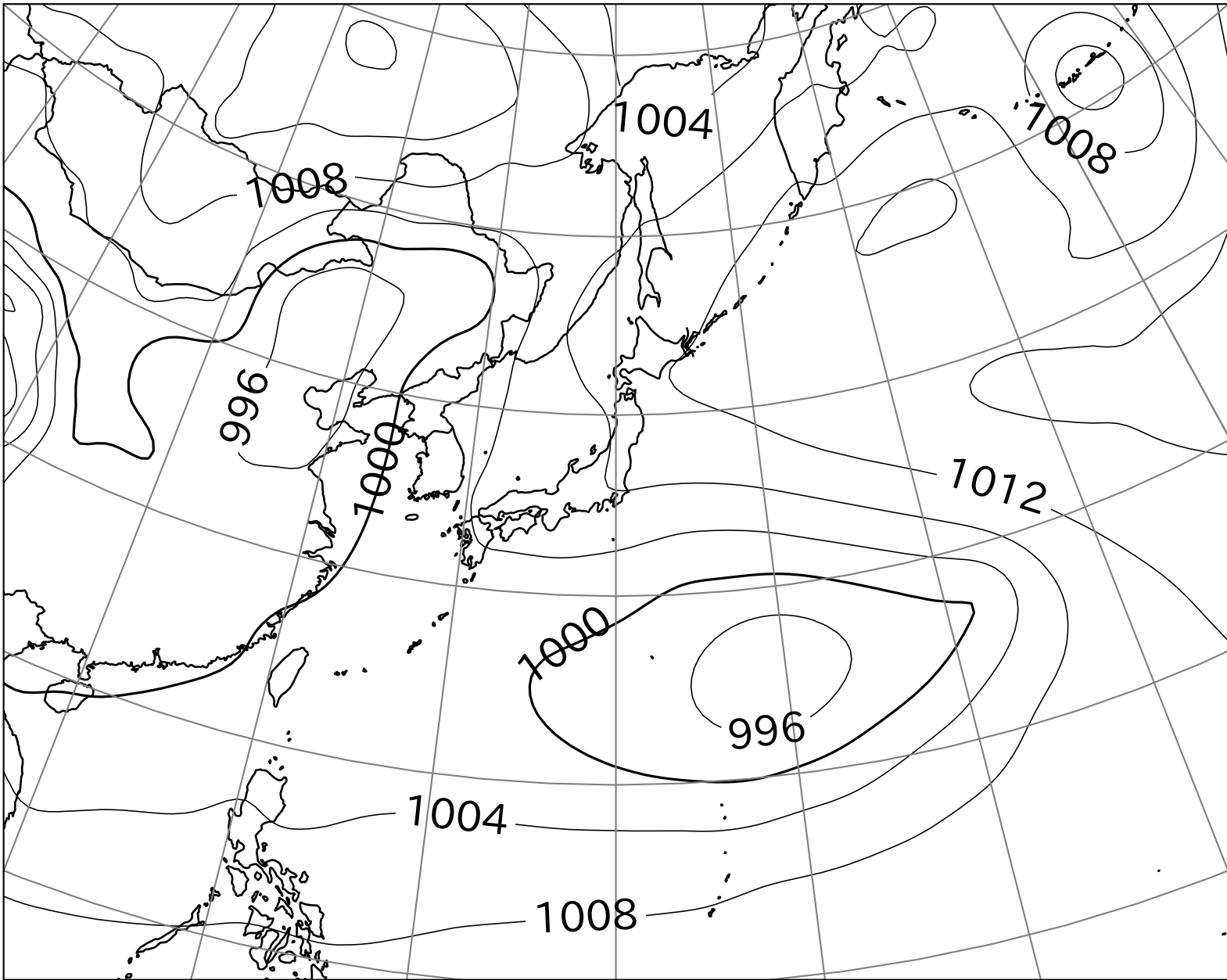
地上天気図
