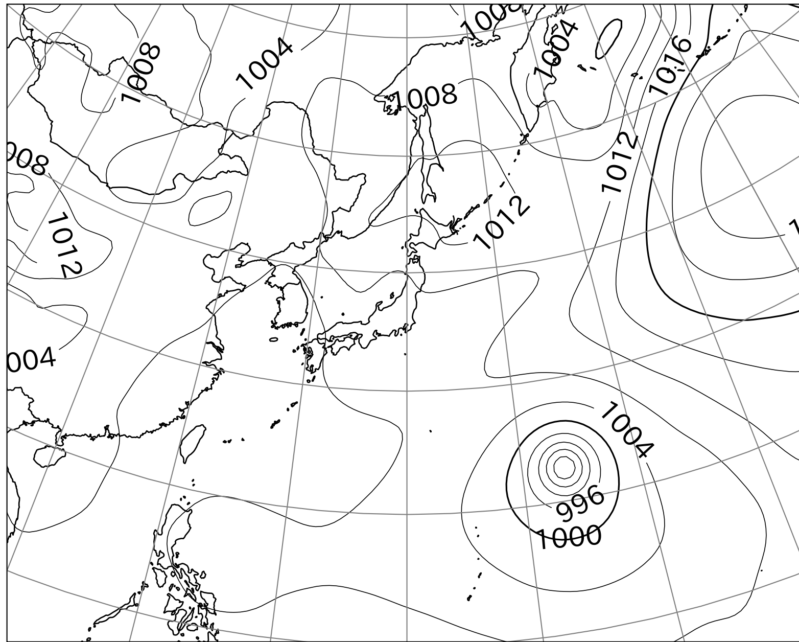
地上天気図
