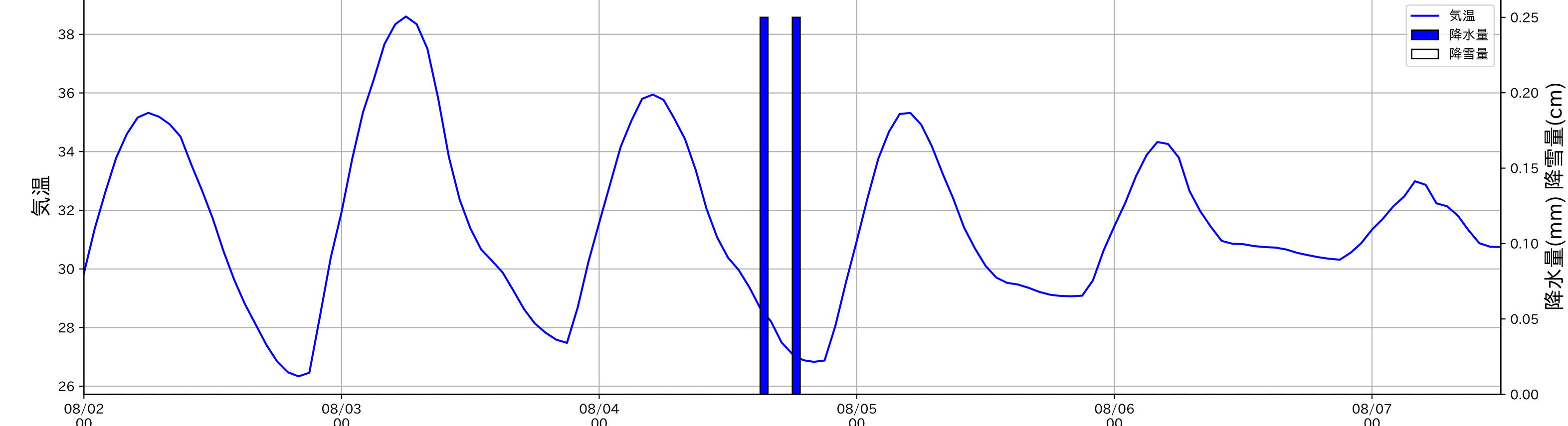
850hpa 気温と高度
