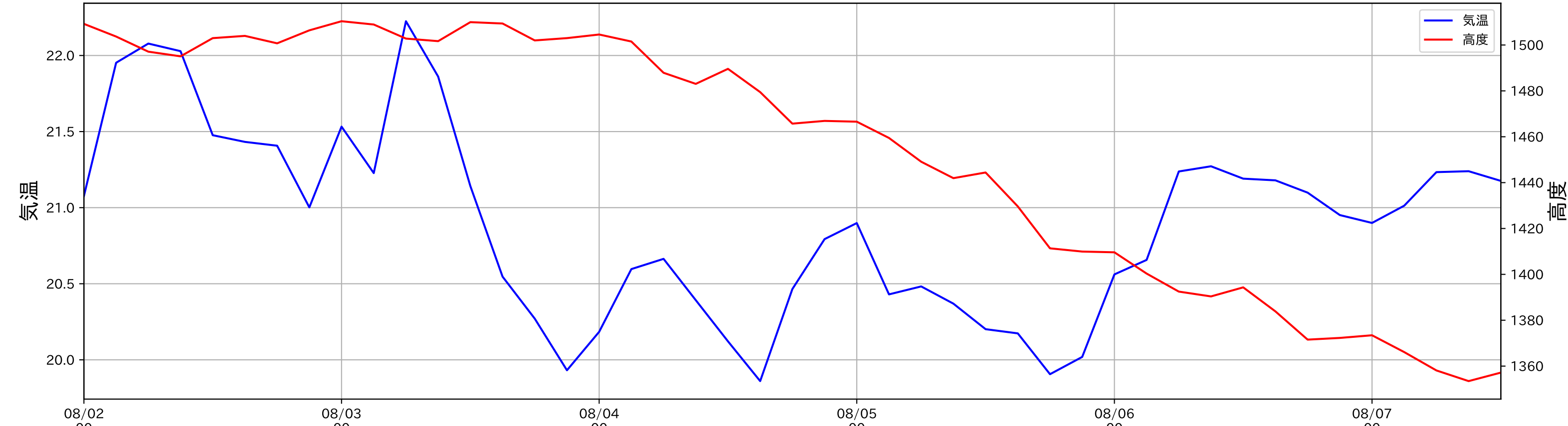
500hpa 気温と高度
